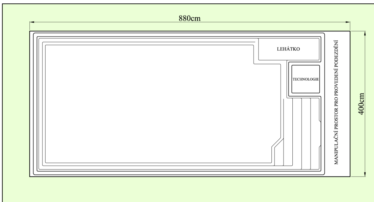
půdorys výkopu
