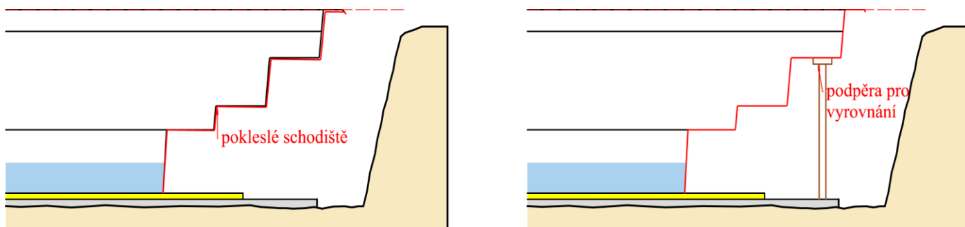
ilustrační obrázek - v případě pokleslého schodiště je nutné toto vyrovnat pomocí podepření lavice
