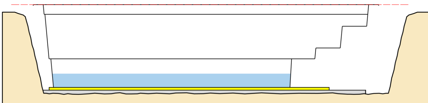
kontrola rovinnosti límce - korekce v případě pokleslého límce se provádí podepřením a srovnáním daného místa
