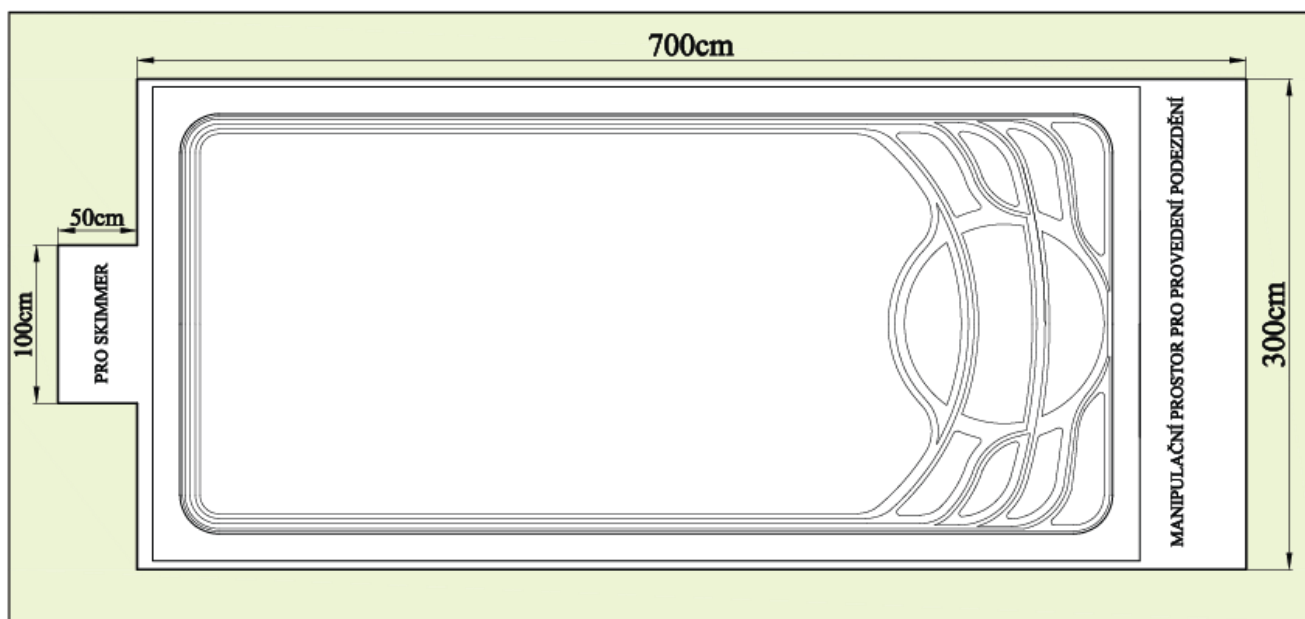
půdorys výkopu
