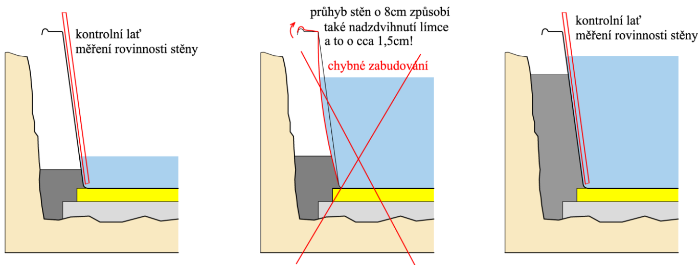
ilustrační obrázek - kontrola rovinnosti stěn ve svislém směru
