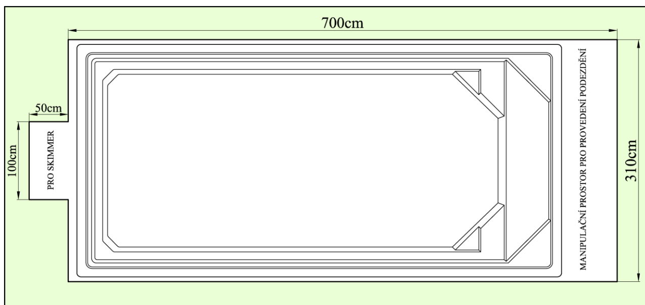
půdorys výkopu
