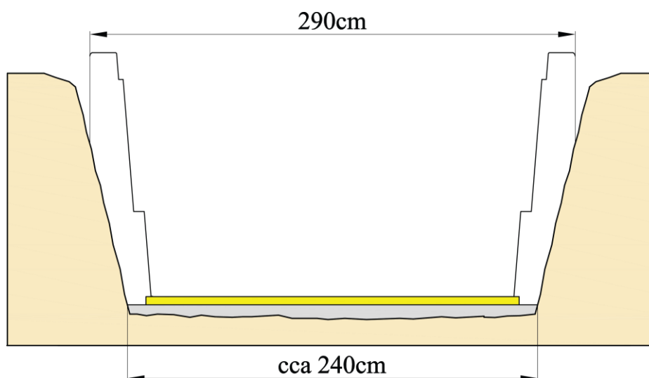
příčný řez výkopem - šířka betonové desky cca 240cm
