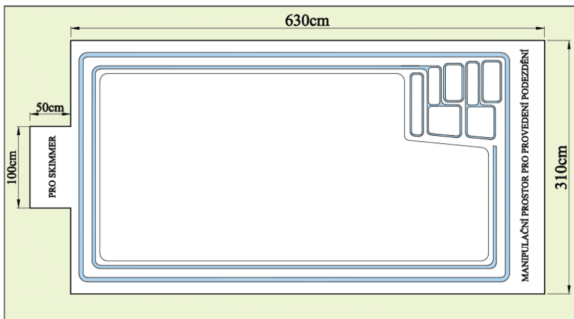
půdorys výkopu
